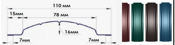
Евроштaketник
